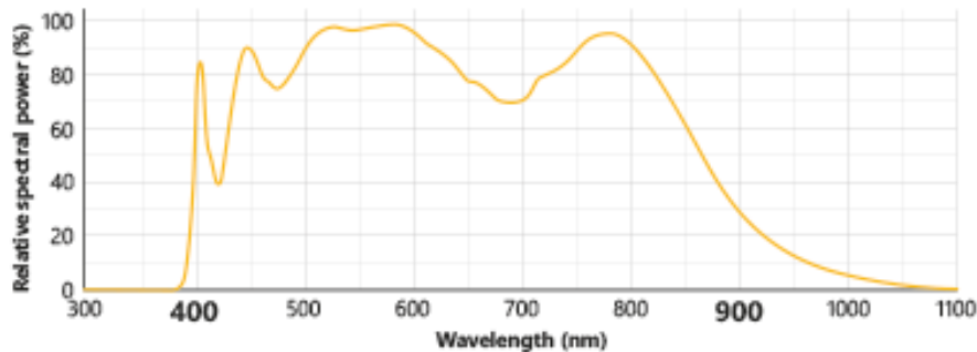
Spectrum of the hyperspectral LED « Visible-NIR »
